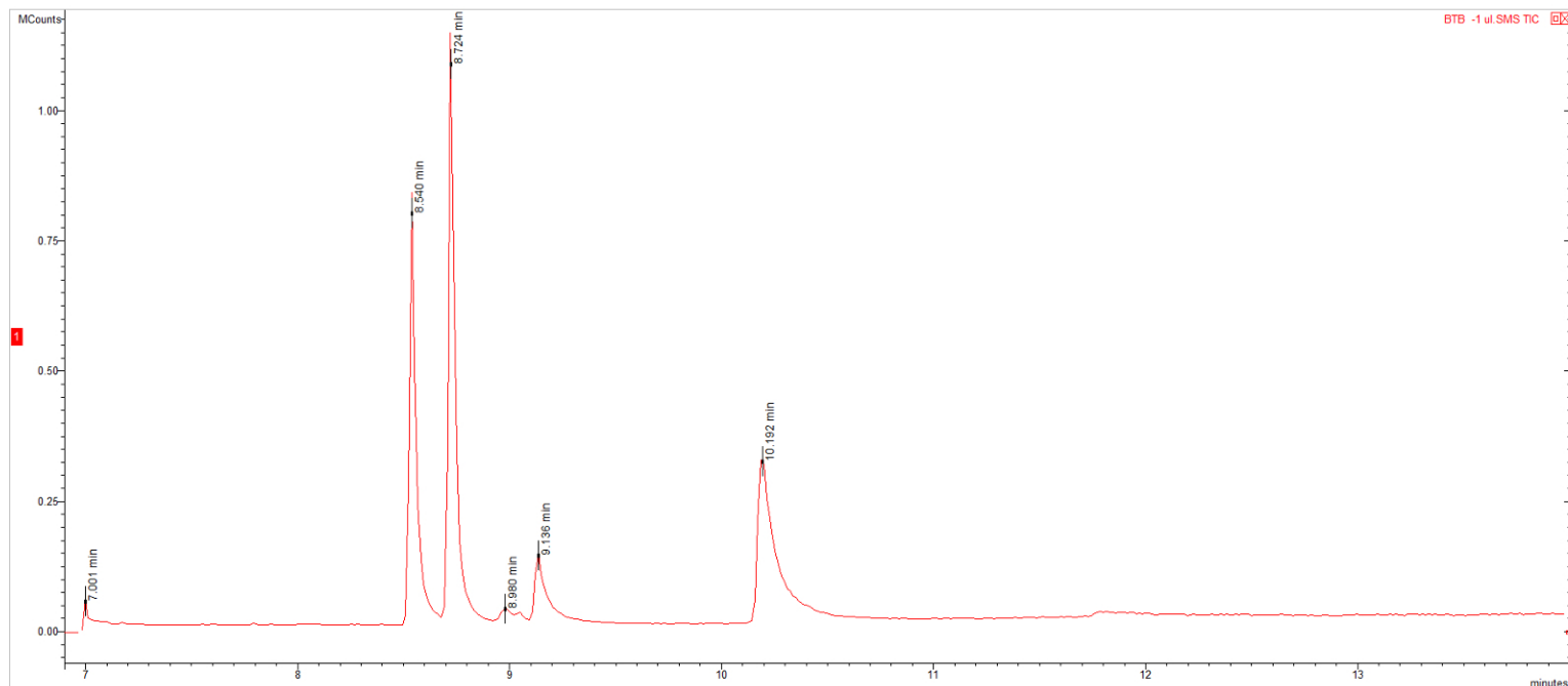
Rys. 1 Widmo masowe dla badanego produktu BTB Man
